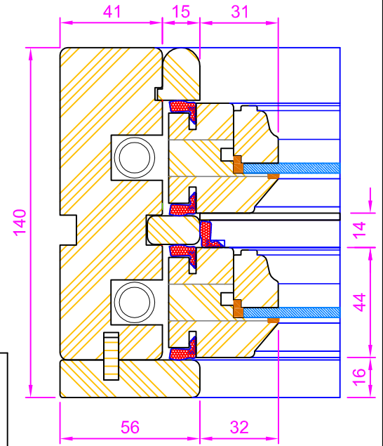
Section B-B (Dwg.No. 3006)
