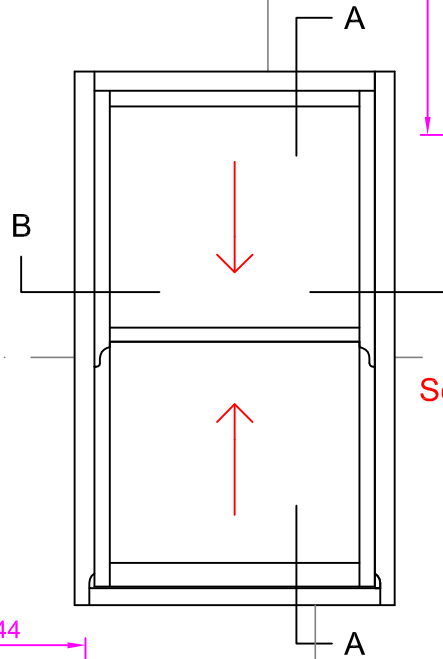
Section A-A (Dwg.No. 3004)
