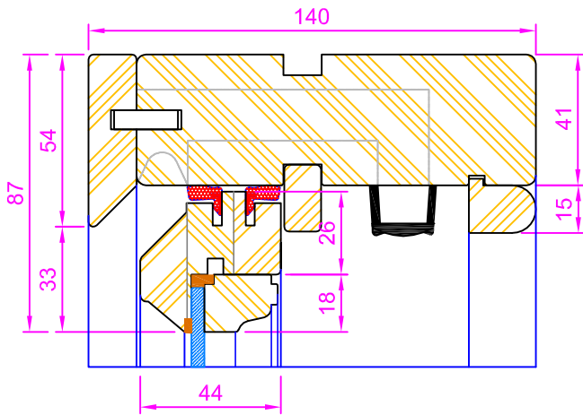
Section A-A (Dwg.No. 3003)
