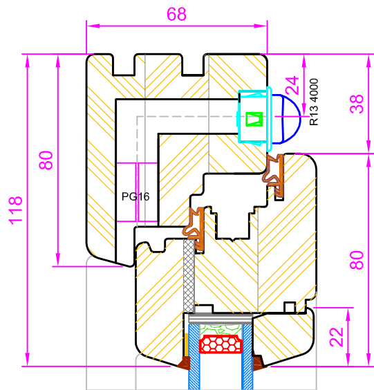
Section A-A (Dwg.No. 0013)
