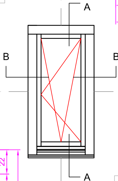
Section A-A (Dwg.No. 0016)
