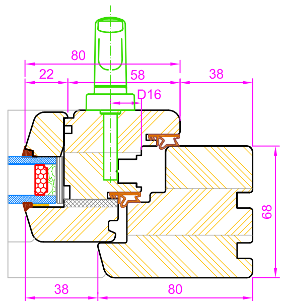
Section B-B (Dwg.No. 0015)
