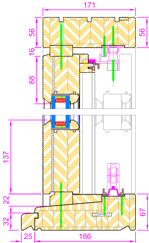
F-F (Dwg.No. 1403 & 1410)
