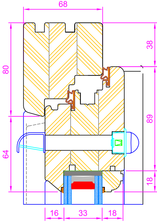
Section A-A (Dwg.No. 2110)
