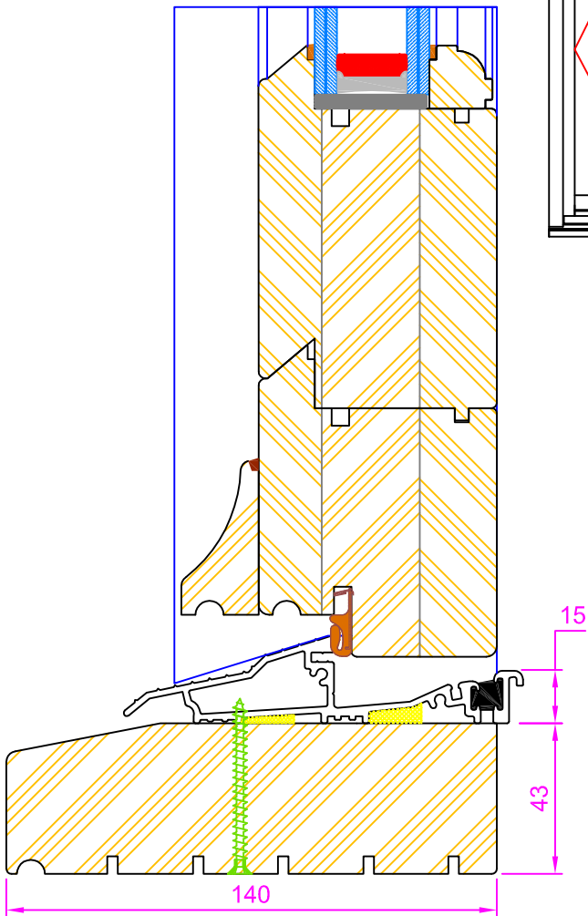
Section A-A (Dwg.No. 2119)
