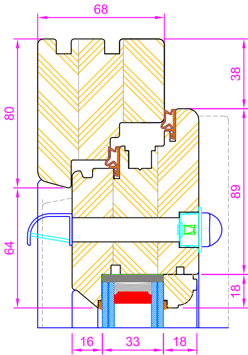
Section C-C (Dwg.No. 2119)
