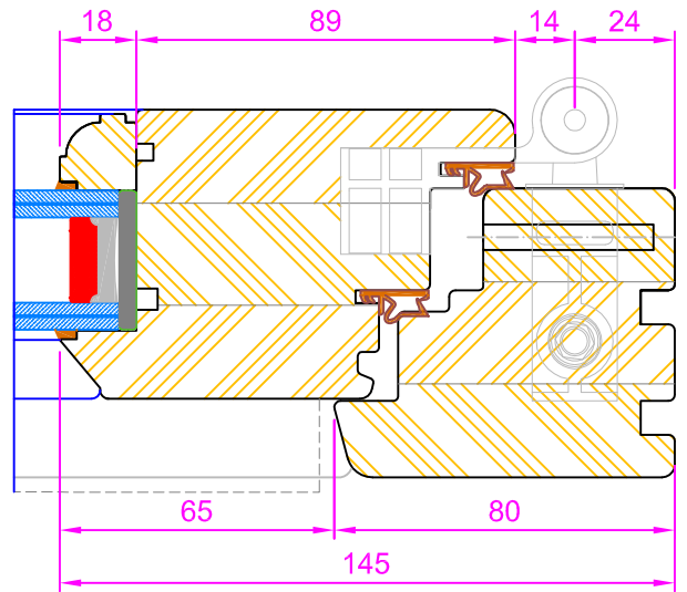
Section B-B (Dwg.No. 2111 mirr'd)
