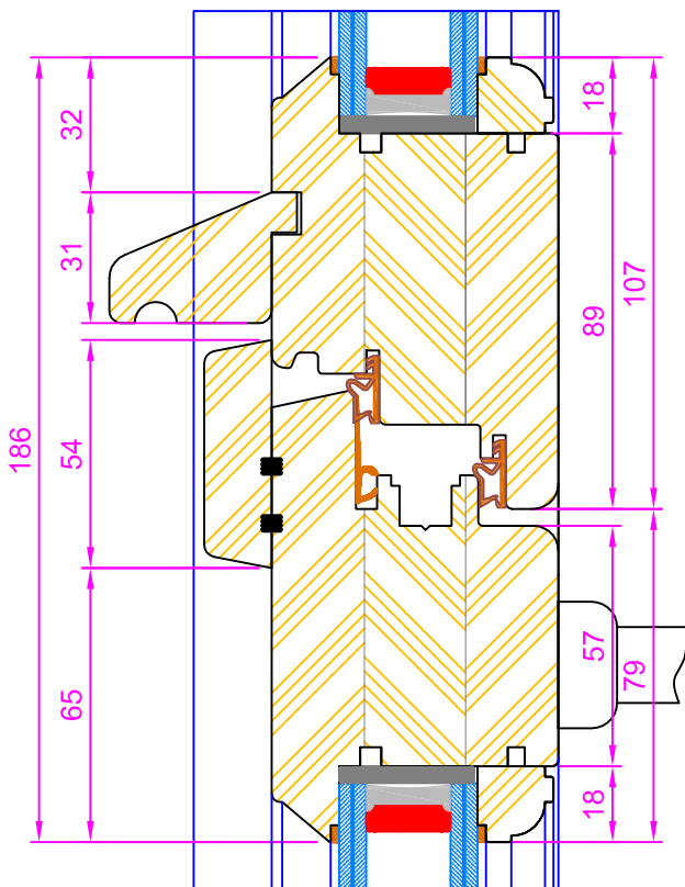
Section C-C (Dwg.No. 2119)
