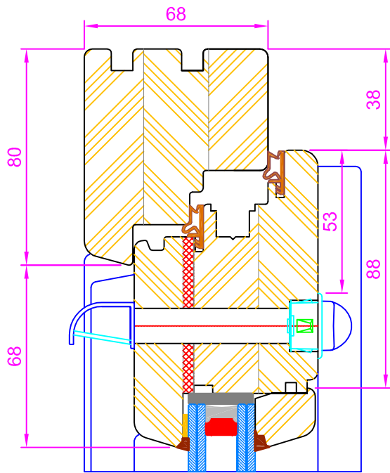
Section A-A (Dwg.No. 1312)
