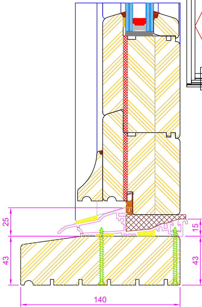
Section A-A (Dwg.No. 1312)
